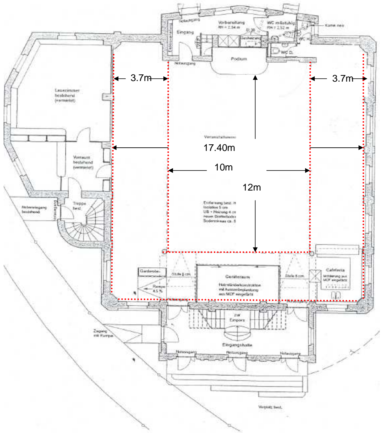
Kirchenarundriss
